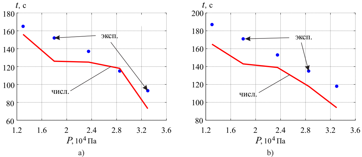
Рис. 6. Время осаждения дисперсной фазы в зависимости от амплитуды волны давления при различных частотах в эксперименте [2] (точки) и полученные из расчета (линия): а) \omega = 158 Гц; б) \omega = 160.66 Гц
