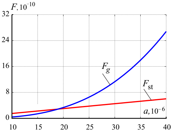
Рис. 1. Сравнение величины силы Стокса F_{st} при некоторой заданной разнице в скорости между частицей и газом и силы тяжести F_g , действующих на отдельную частицу, в зависимости от радиуса частицы a
