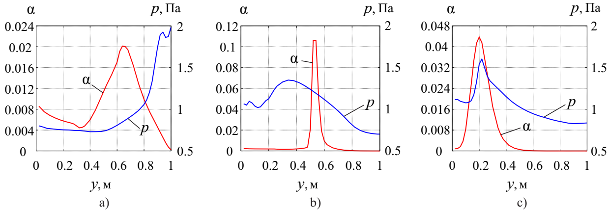
Рис. 4. Распределение концентрации дисперсной фазы \alpha_2 и давления p в моменты времени t = 30 \text{ с} (а), t = 60 \text{ с} (b) и t = 90 \text{ с} (с)
