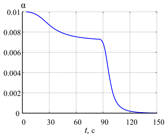
Рис. 5. Изменение средней концентрации дисперсной фазы \bar{\alpha}_2 в расчетной области с течением времени
