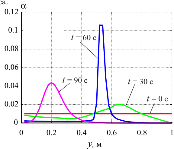
Рис. 3. Изменение концентрации дисперсной фазы \alpha_2 с течением времени
