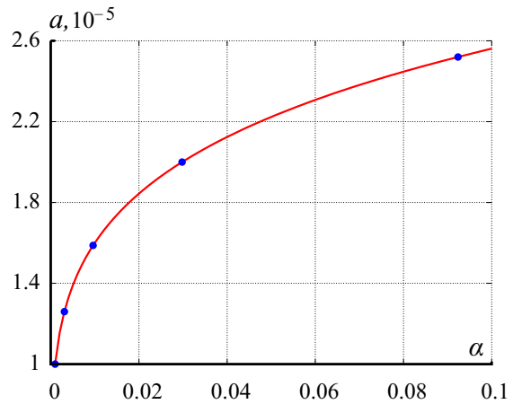
Рис. 2. Зависимость эффективного радиуса \tilde{a} частиц гранулированной фазы от концентрации \alpha_2 ; точками обозначены значения размеров дисперсных частиц при заданных \alpha_i
