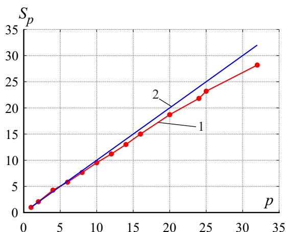
Рис. 7. Зависимость ускорения вычислительного процесса от числа используемых ядер (линия 1); для сравнения приведена линия 2 линейного роста ускорения
