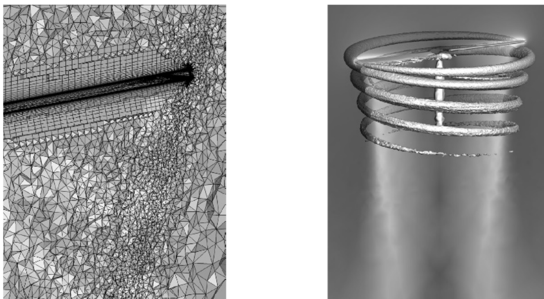
Рис. 4. Фрагмент неструктурированной сетки (слева), визуализация концевых вихрей несущего винта на режиме висения (справа)
