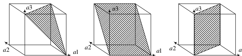
Рис. 4. Логические ограничения на сечения
